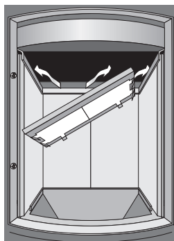
5. Den Halterahmen mit eingelegten Filtern einsetzen
