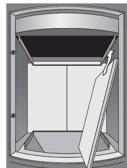
3. Feuerraumseitenwand einsetzen
