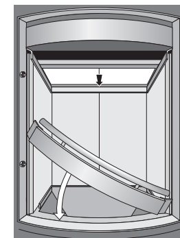
6. Stehrost einsetzen
