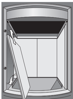
4. Feuerraumseitenwand einsetzen
